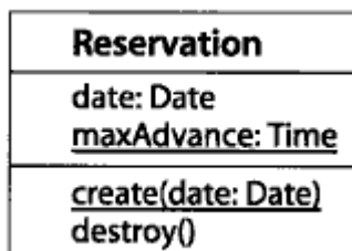
图 13-139 类级作用域的属性 and 操作
