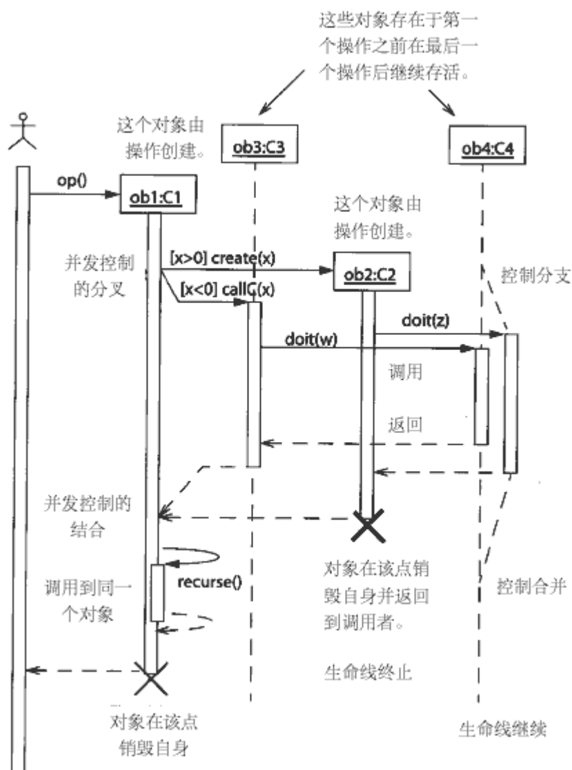
图 13-162 显示了顺序图上的控制过程流。当为控制过程流建模时，对象产生对一个调用的控制直到返回。调用以实心箭头表示。调用箭头的头部可能激发一个活动或者是一个新的对象。返回以虚线显示。返回箭头的尾部可能结束这个活动或者对象。
