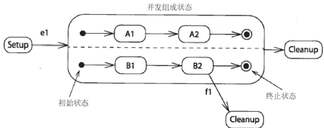
图 13-59 复杂转换（分支，结合）
