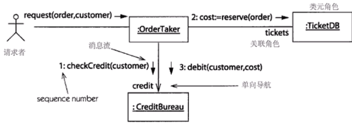
图 8-3 合作图
