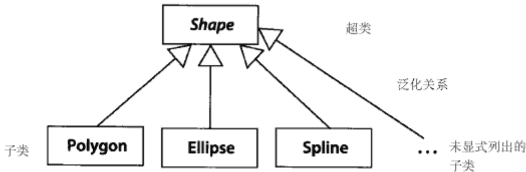
图 13-102 泛化关系
