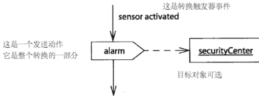
图 13-80 信号发送
