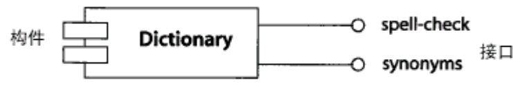
图 9-1 带接口构件
