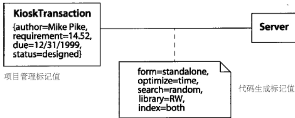
图 11-2 标签值
