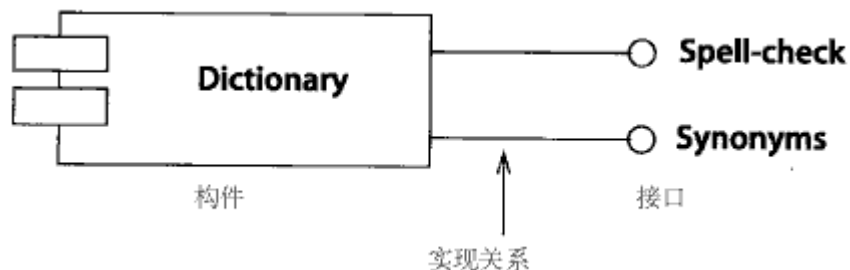
图 13-60 构件
