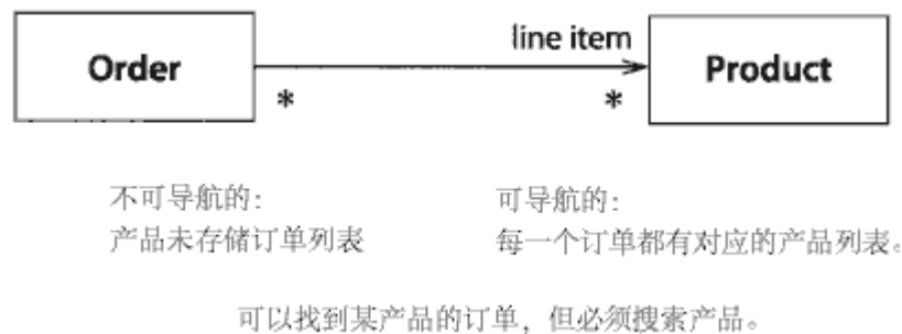
图 13-131 导航性
