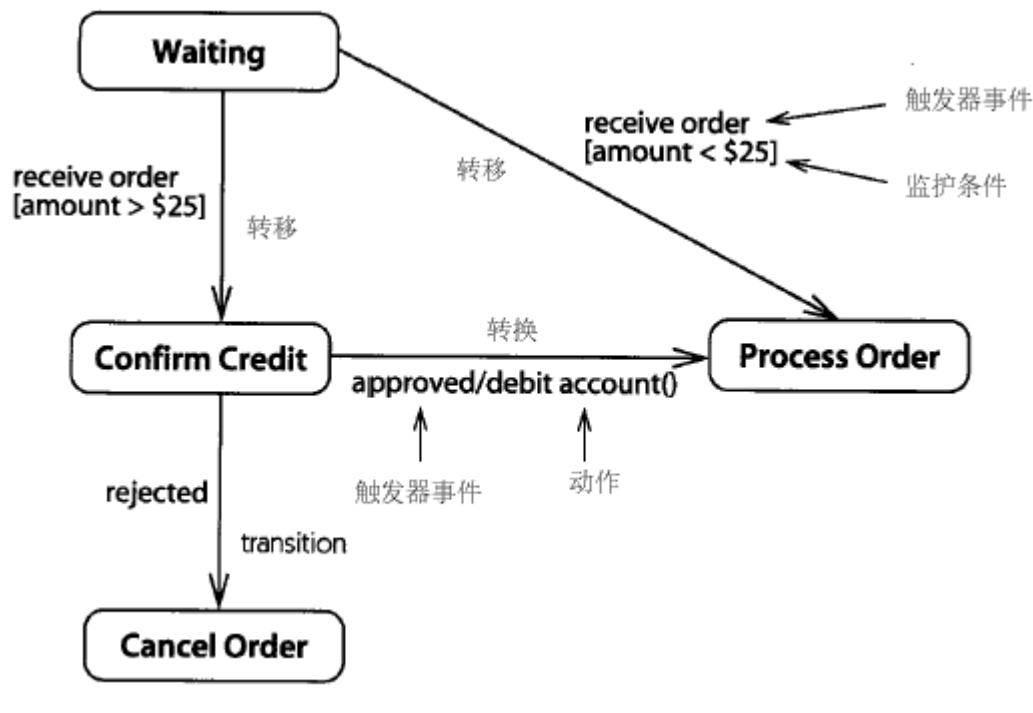
图 6-3 外部转换
