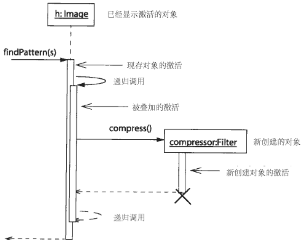
图 13-7 激活
