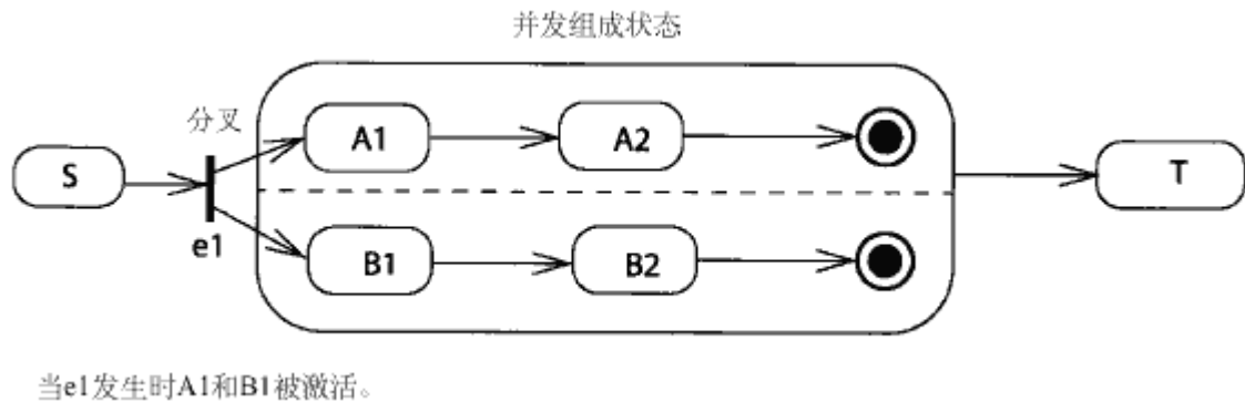
图 13-101 分叉
