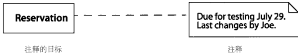
图 13-52 注释
