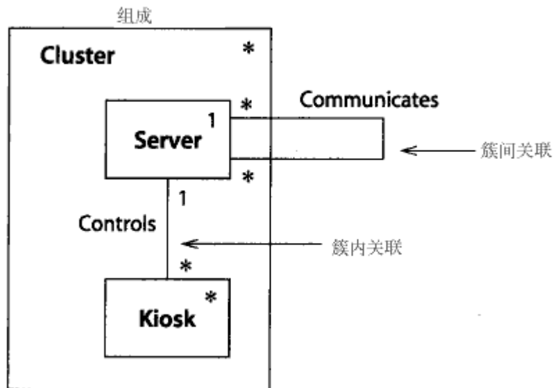
图 13-70 组成之内和之外的关联
