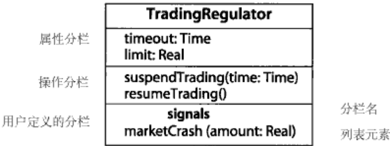
图 13-53 类中命名的分格
