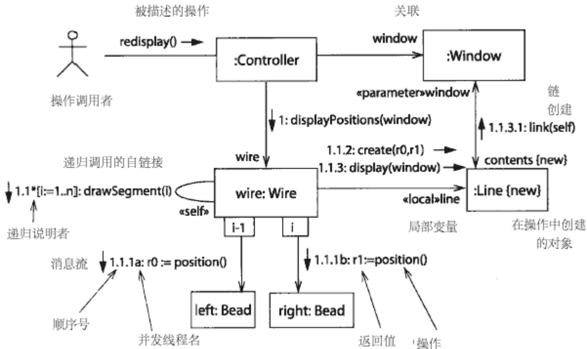
图 13-51 帶有消息流的合作圖
