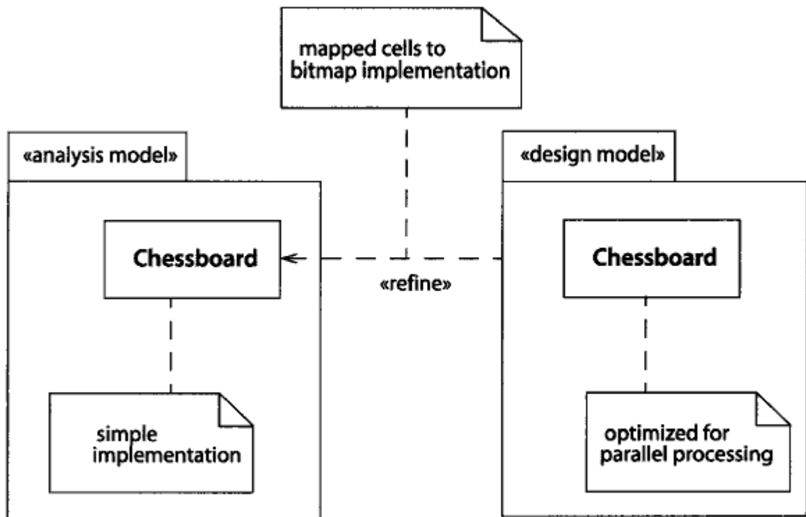
图 13-156 细化
