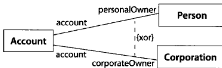
图 13-25 异或关联
