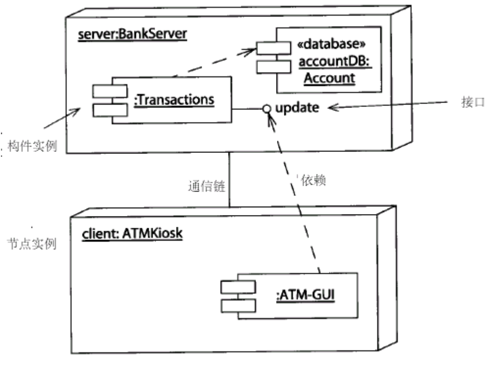
图 9-3 部署图
