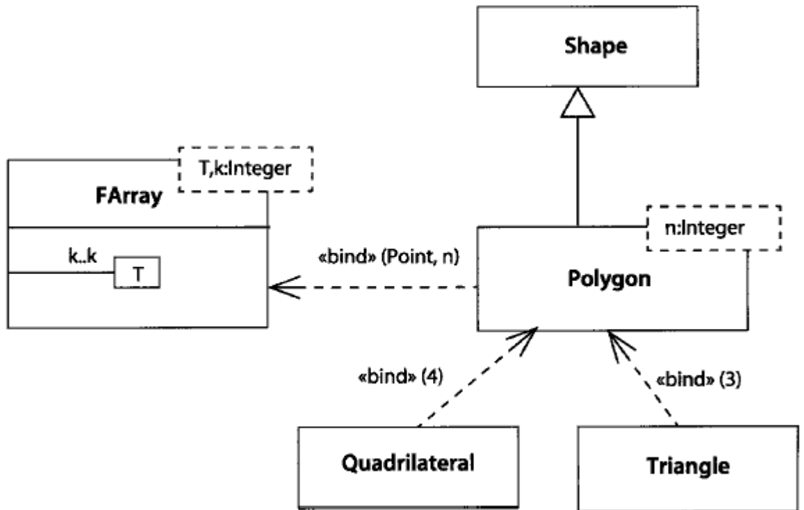
图 13-35 模板再绑定
