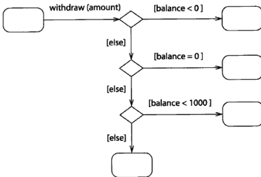
图 13-183 是一个示例。
