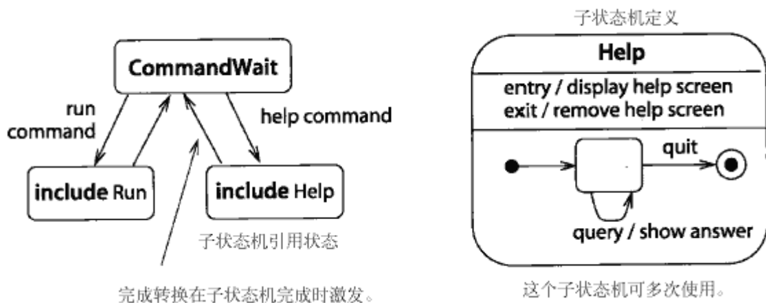
图 13-167
