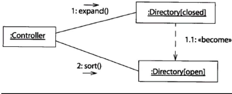
图 8-4 变成流
