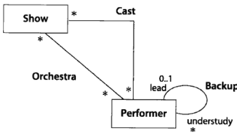
图 13-22 关联
