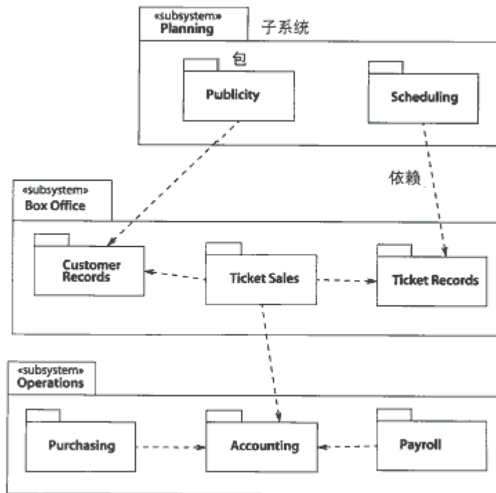
图 3-10 包
