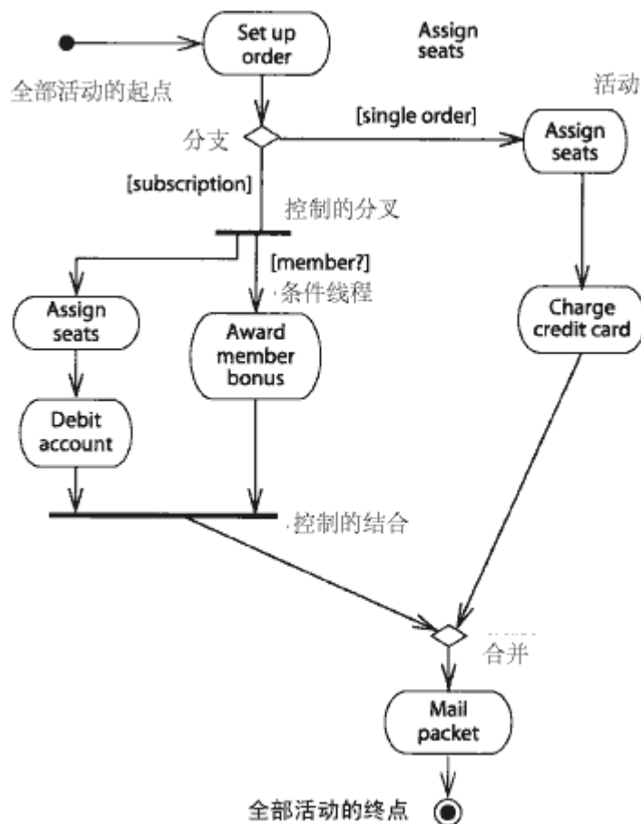
图 13-12 活动图
