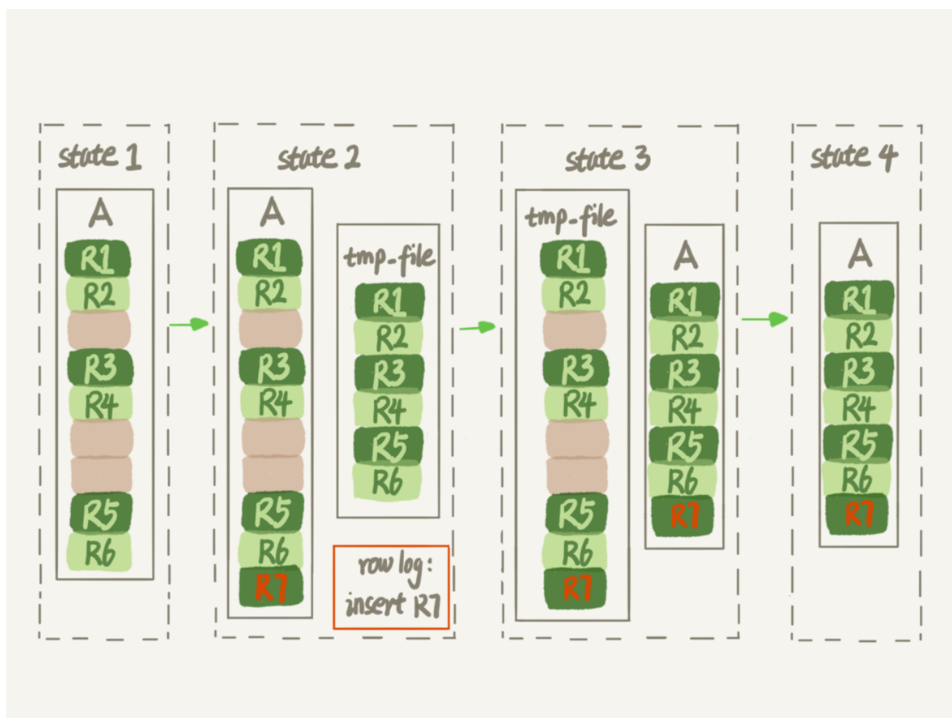
图 4 Online DDL
