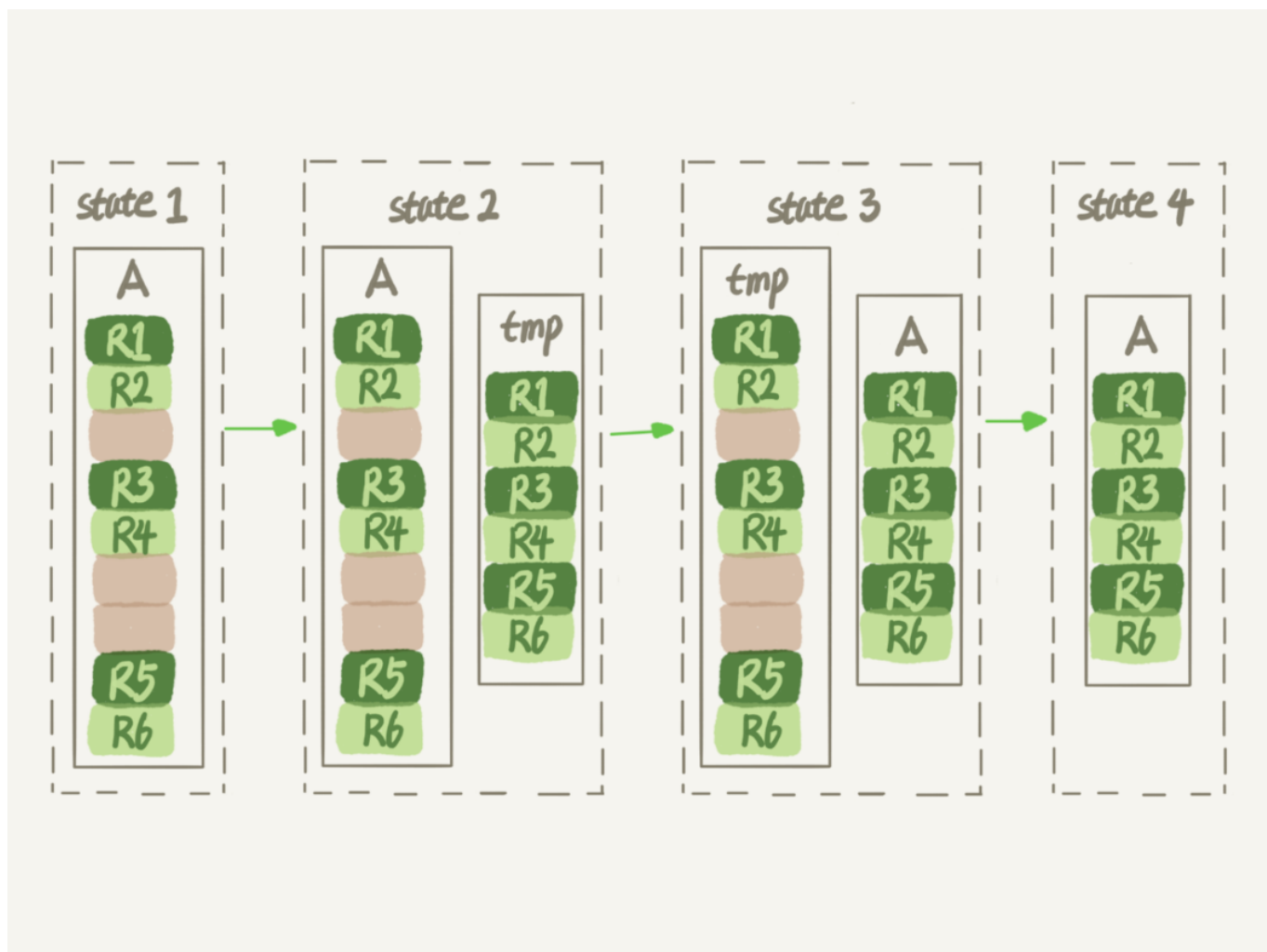
图 3 改锁表 DDL
