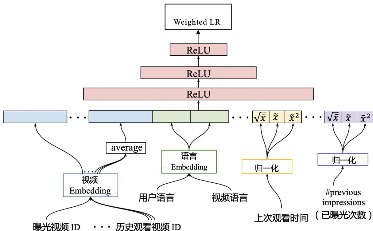
图3 YouTube的深度学习排序模型的架构
