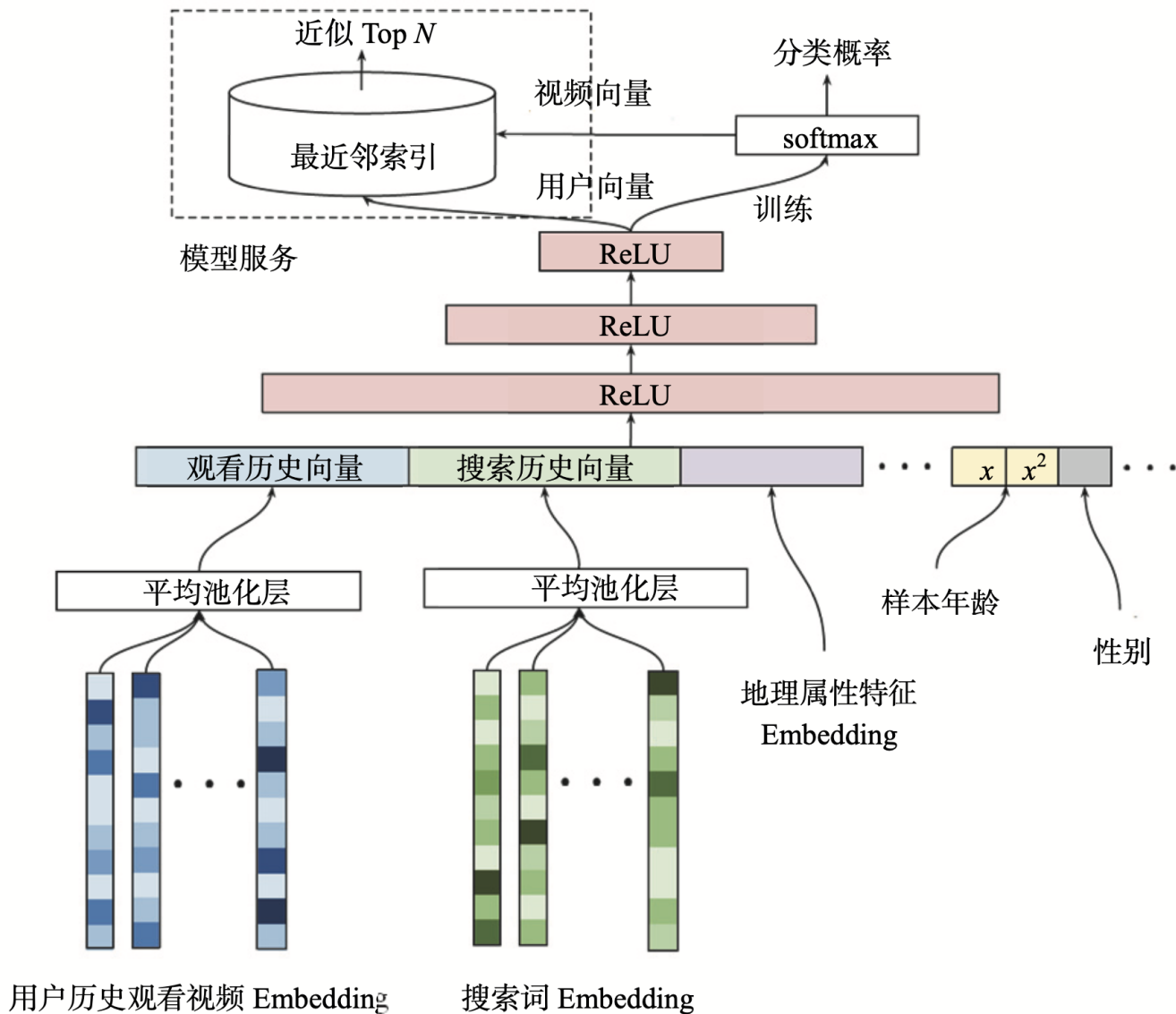
图2 YouTube候选集生成模型架构
