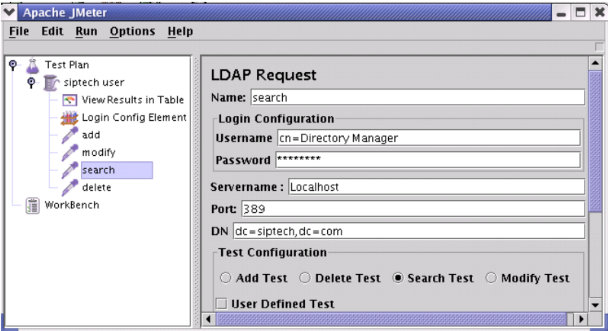
图 9.4.4 Inbuilt-Search Test LDAP 请求
