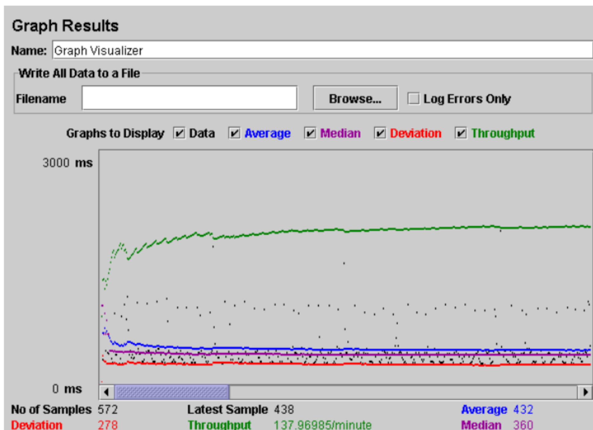
图 5.7. 图像结果监听器
