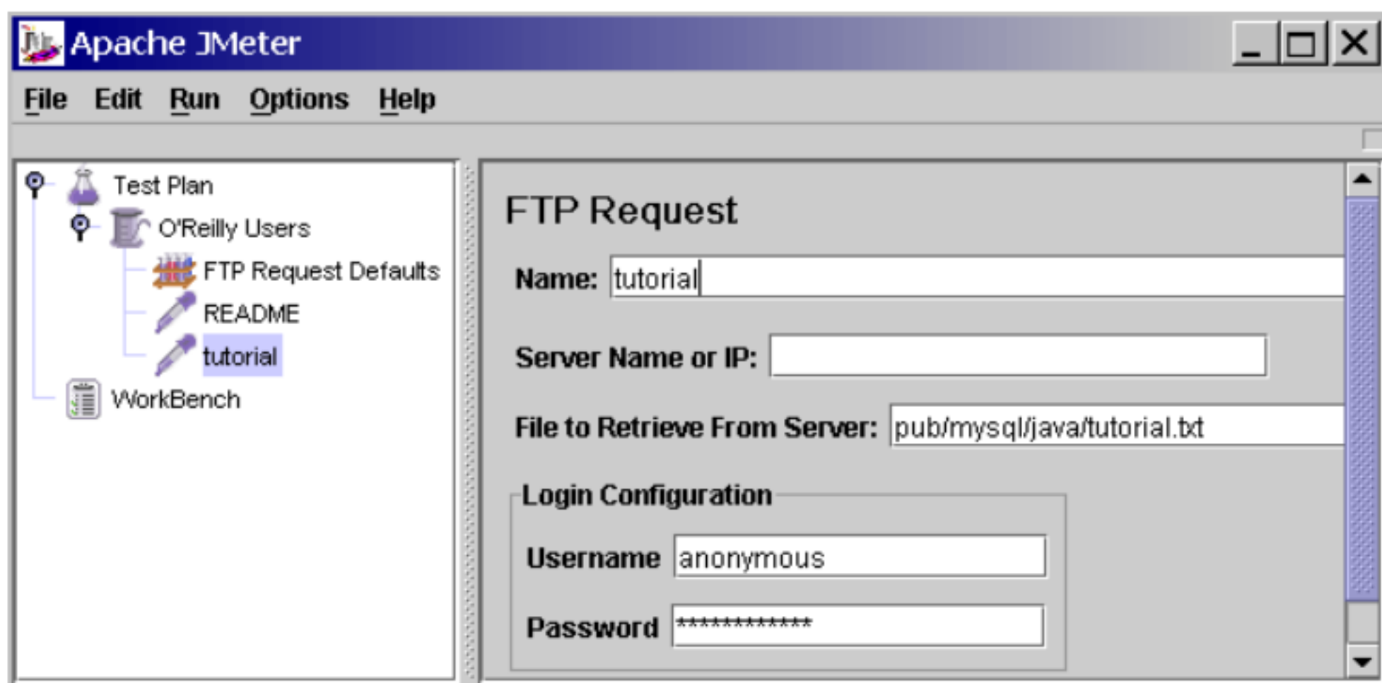
图 8.6 O'Reilly mSQL java tutorial 文件的 FTP 请求
