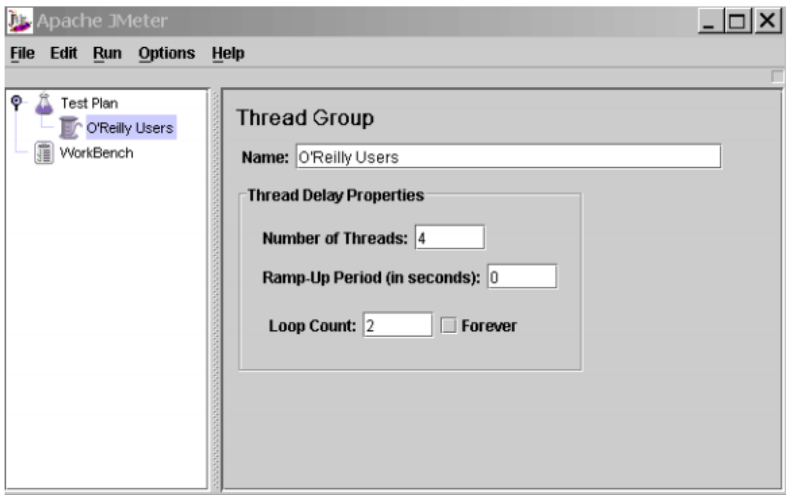
图 8.2 O'Reilly Users 线程组
