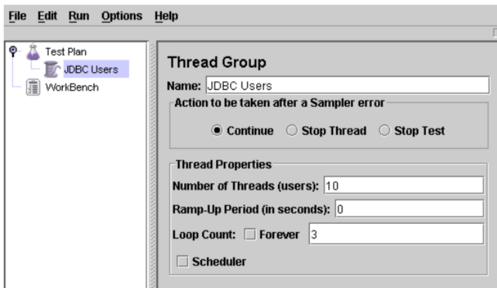
图 7.2 为完整的 JDBC Users 线程组。
