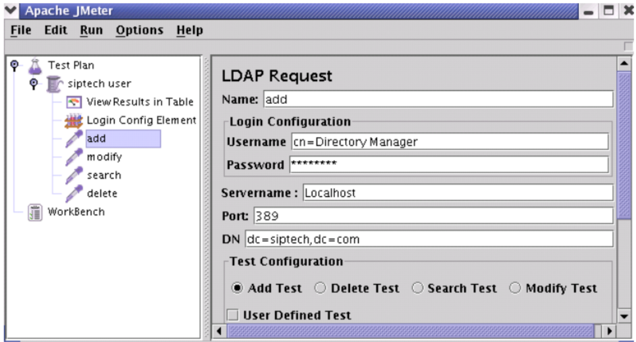
图 9.4.1 Inbuilt Add test LDAP 请求
