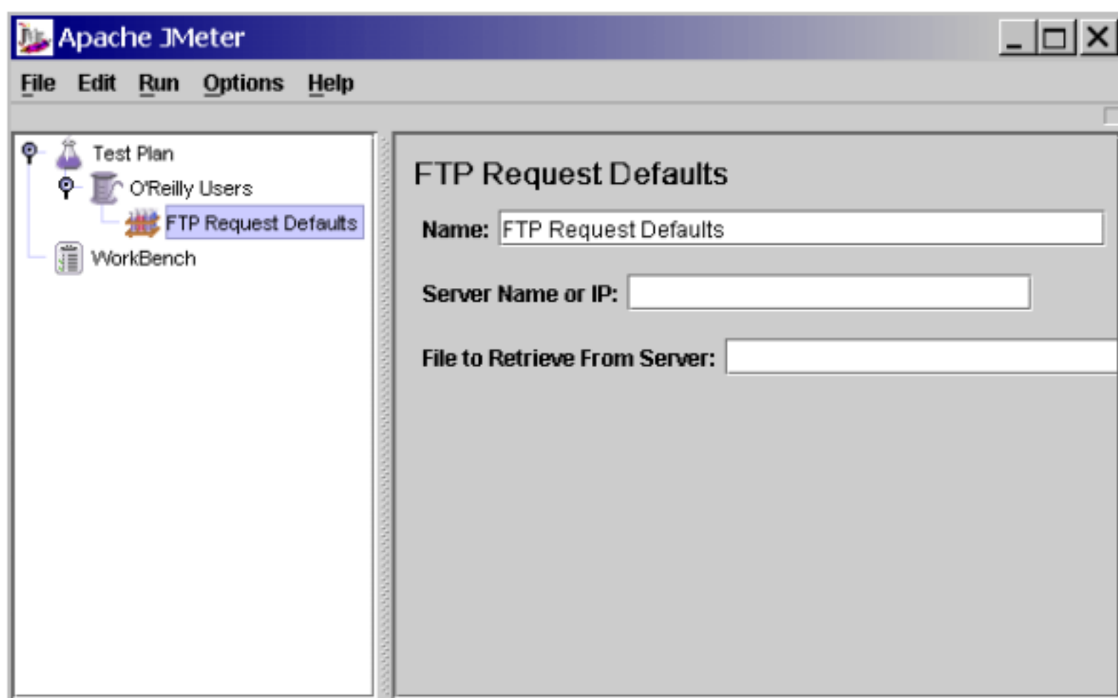
图 8.3 FTP 默认请求
