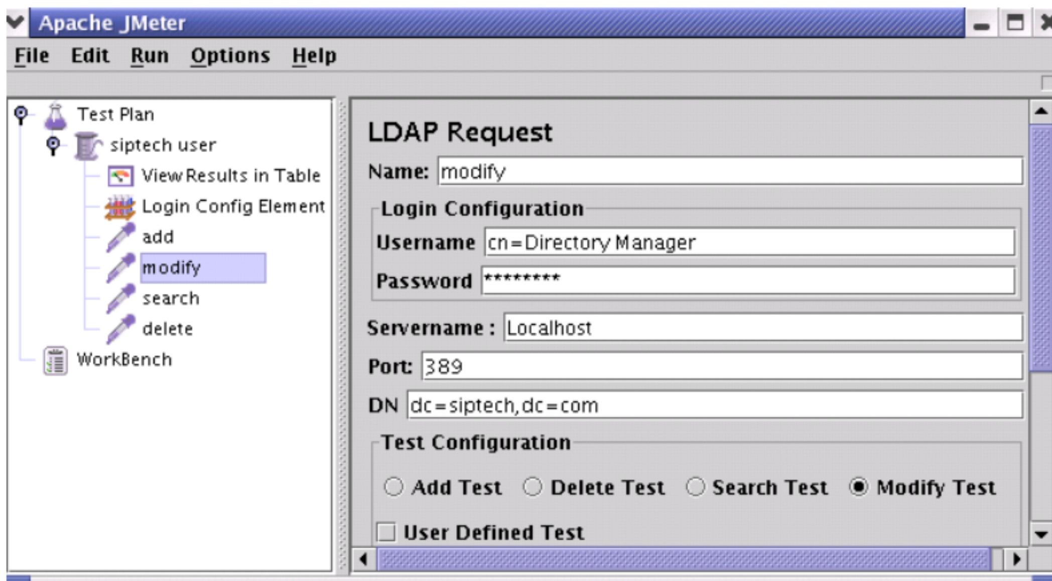
图 9.4.2 Inbuilt Modify test LDAP 请求
