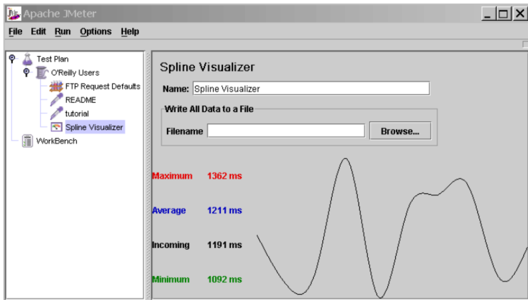
图 8.7 Spline Visualizer 监听器
