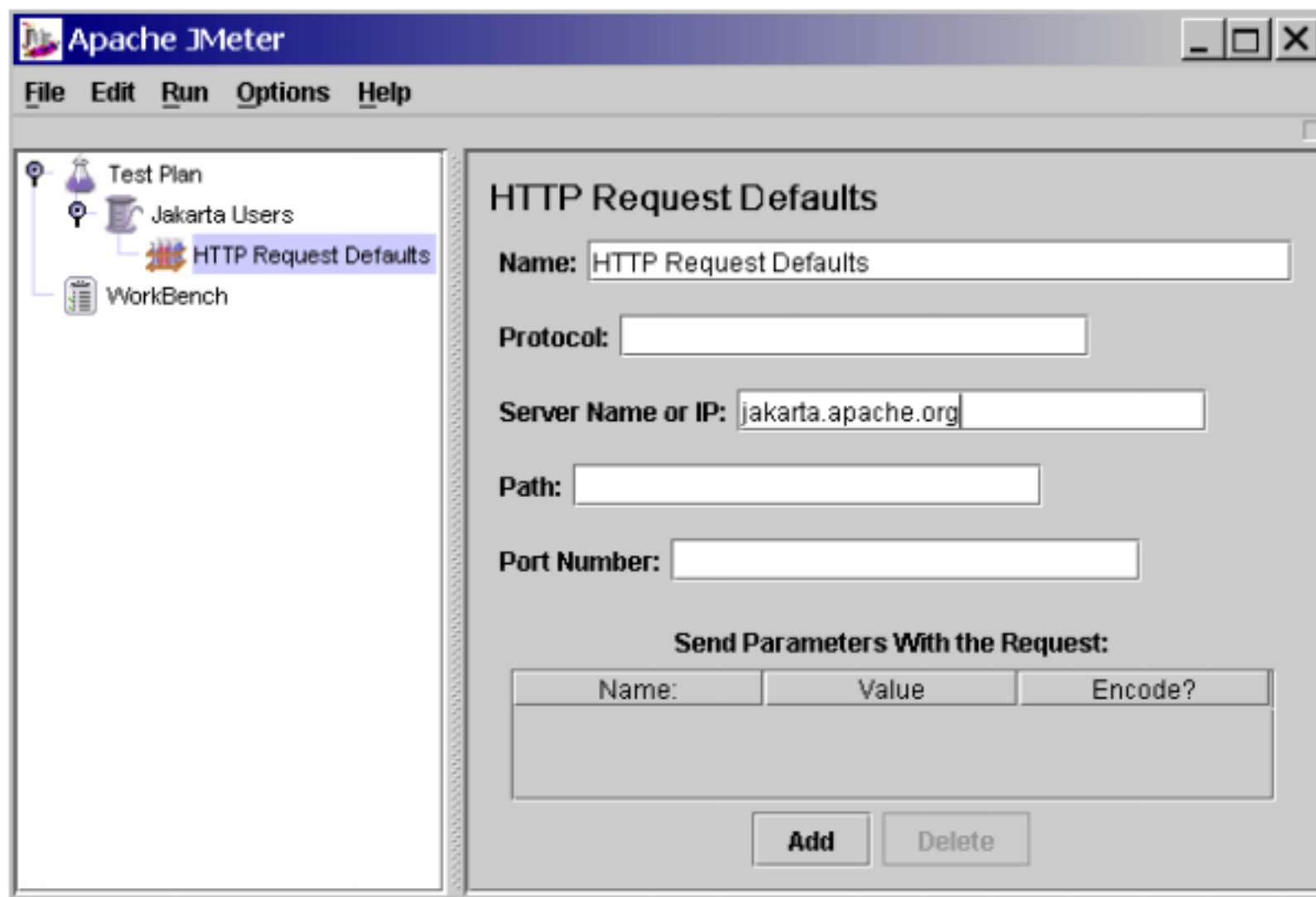
图 5.4. 测试计划的 HTTP 默认值
