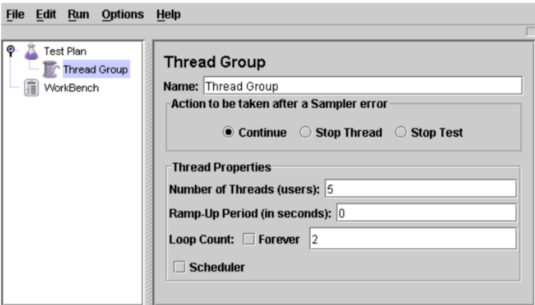
图 10.2 Jakarta Users 线程组
