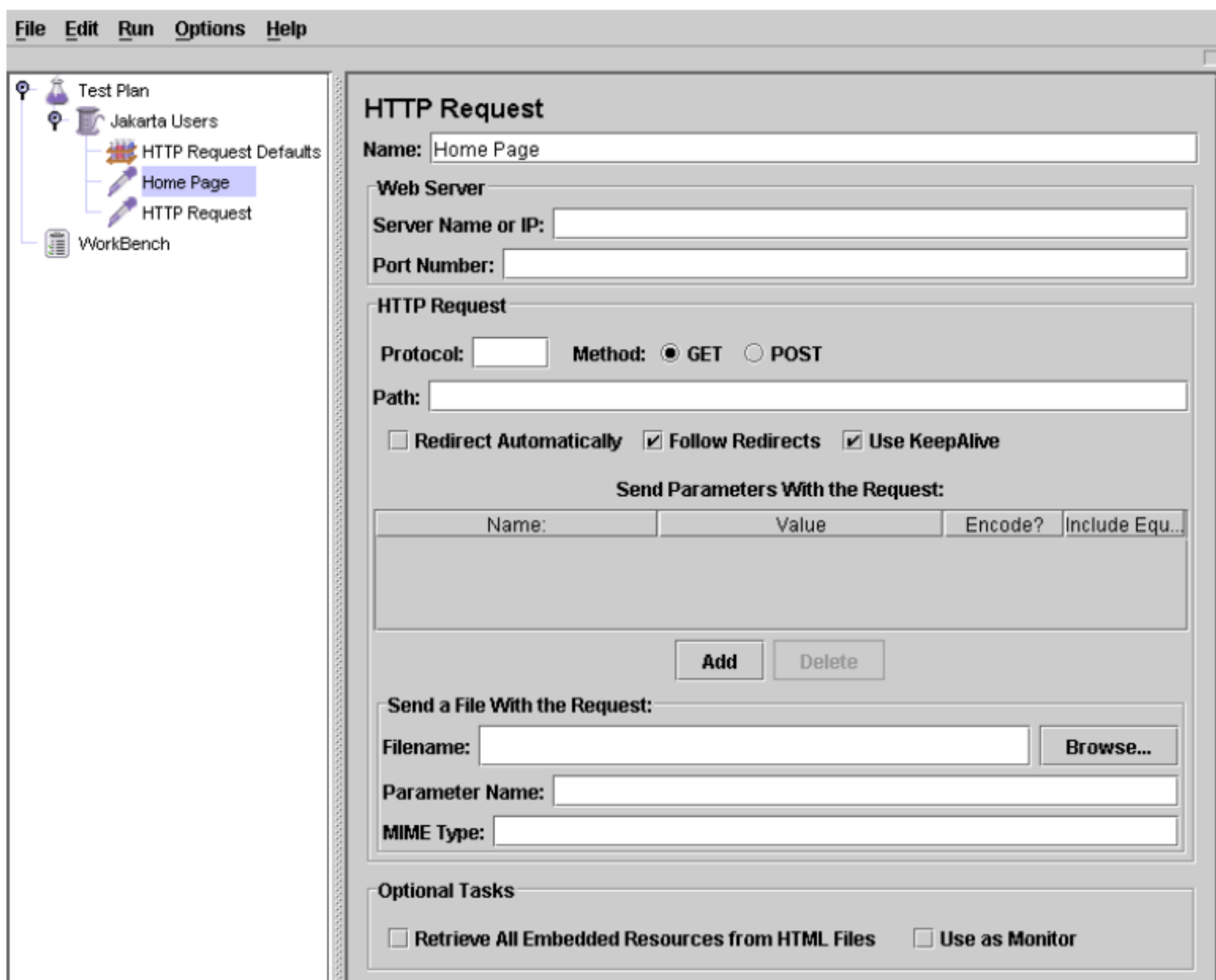
图 5.5. Jakarta 首页的 HTTP 请求
