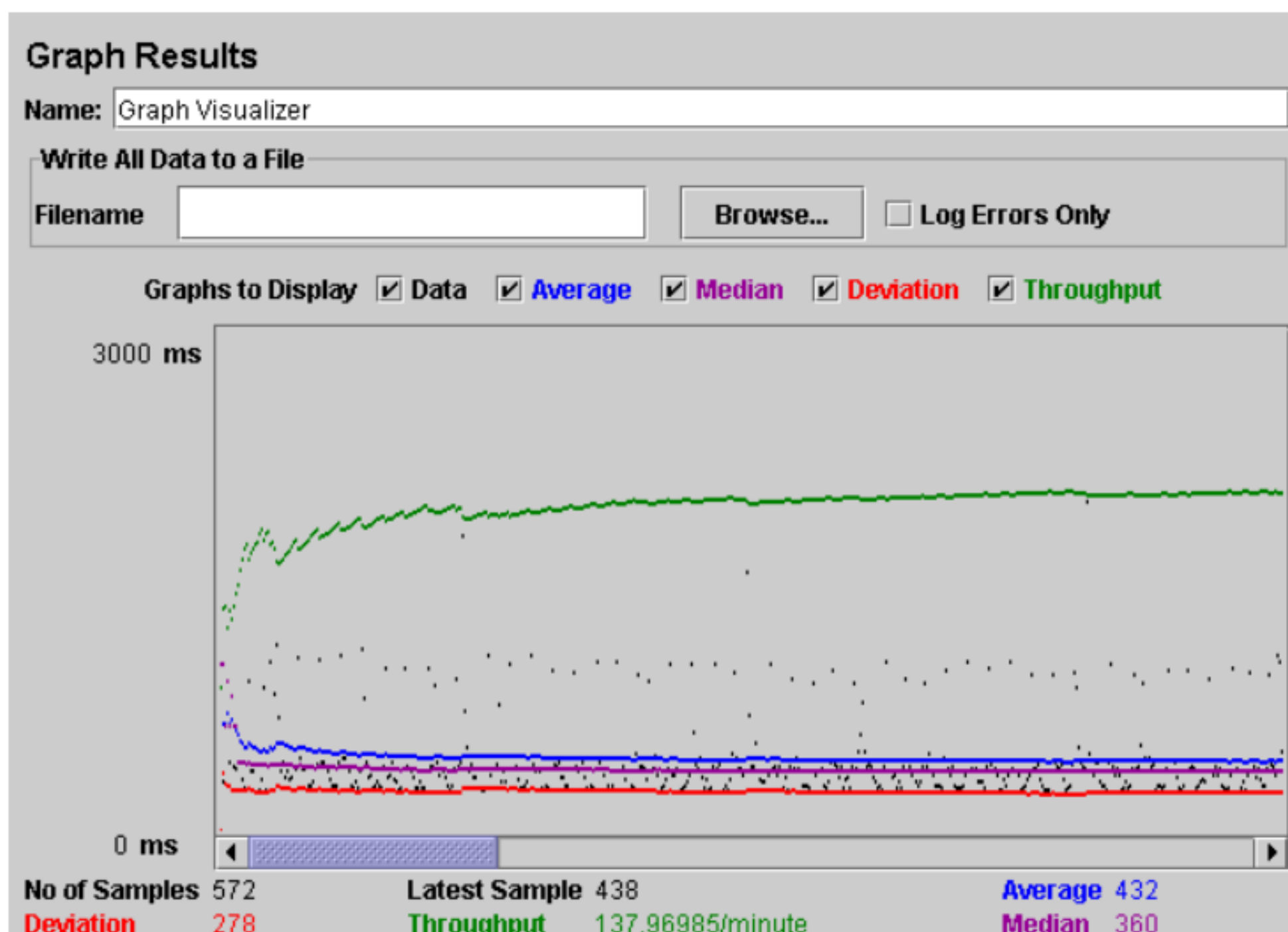
图 12.4 Graph Results 监听器
