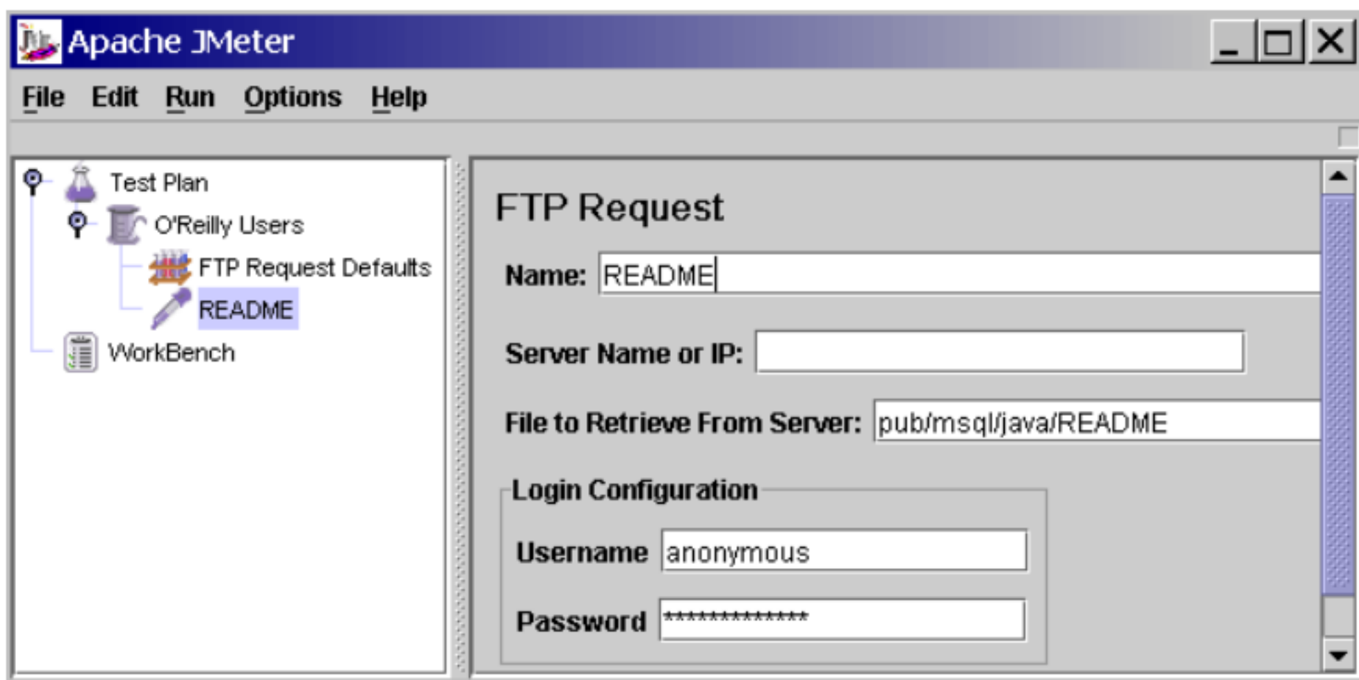
图 8.5 O'Reilly mSQL java README 文件的 FTP 请求
