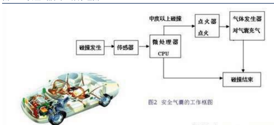
图 18：安全气囊的工作原理图
