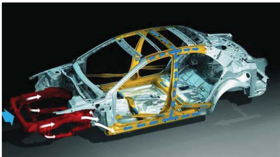
图 20: 防撞车身结构碰撞吸能示意图
