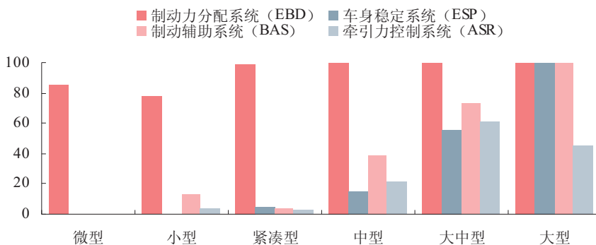
图 8: 我国制动系统相关主动安全领域各级别车型的装备率
