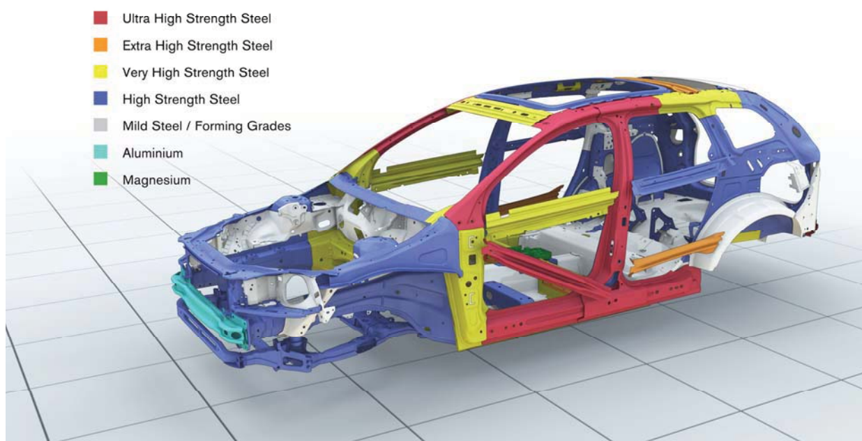
图 21：沃尔沃 XC60 的车身结构，红色为极高强度钢
